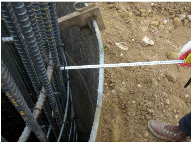
P2 현장타설말뚝 철근망 철근피복두께측정
